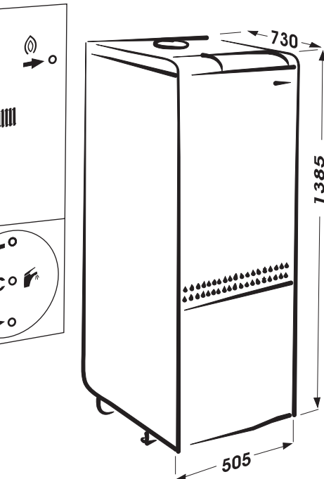
Котлы KLZ С – выход для подключения системы рециркуляции ГВС
