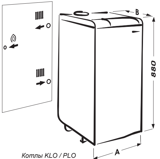
Котлы KLO / PLO
